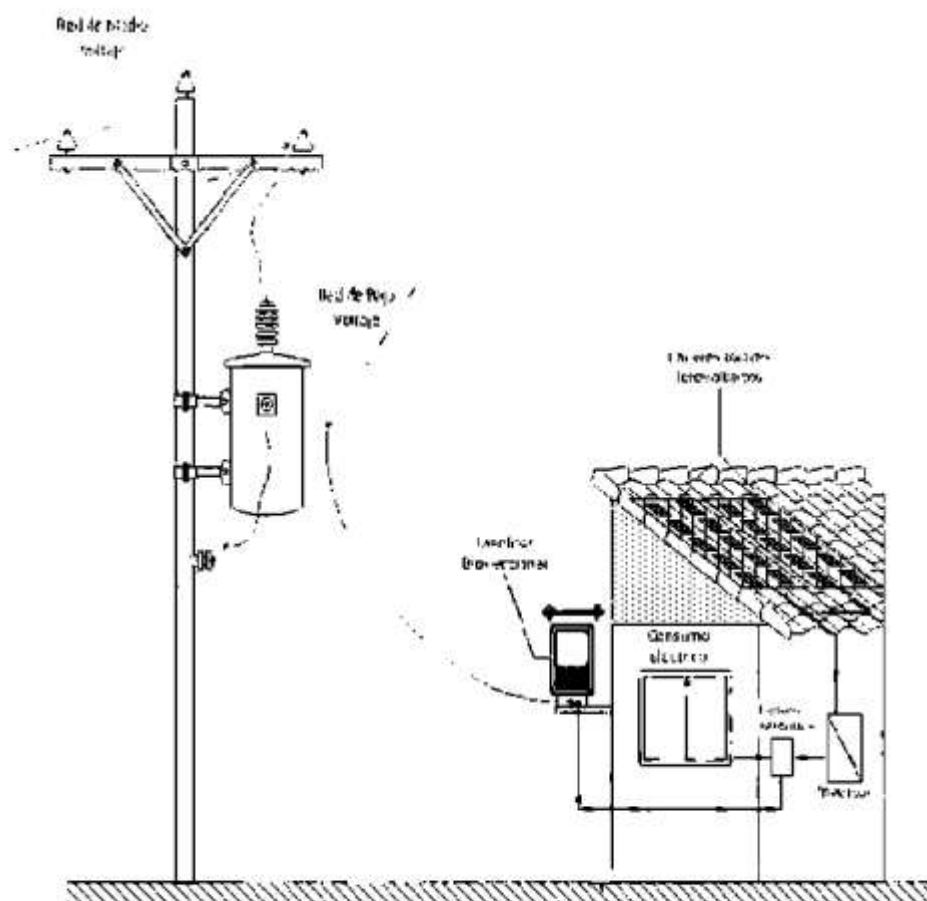
Figura 1. Esquema de instalación del \mu SFV
